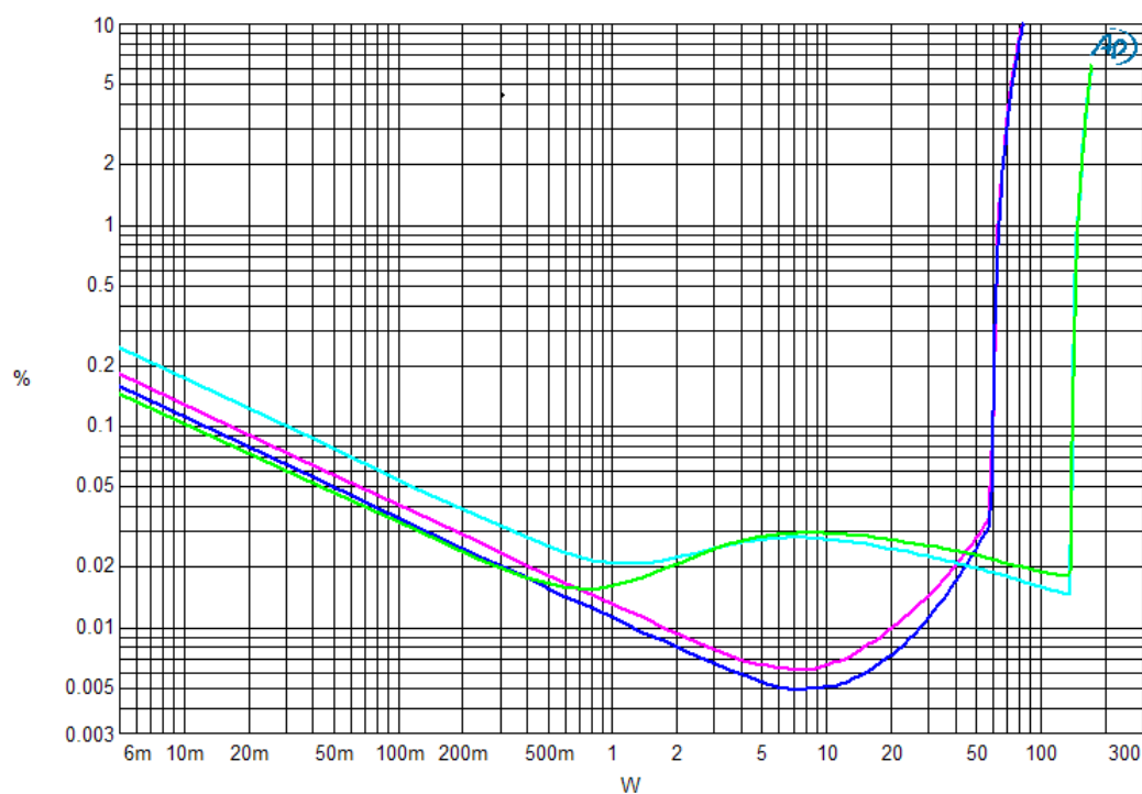
T.H.D + N rispetto alla potenza di uscita su 8Ω classe A e classe AB, 22kHz banda di misura. (BLU ch. SX classe A, ROSA ch. DX classe A, VERDE ch. SX classe AB, CELESTE ch. DX classe AB)
