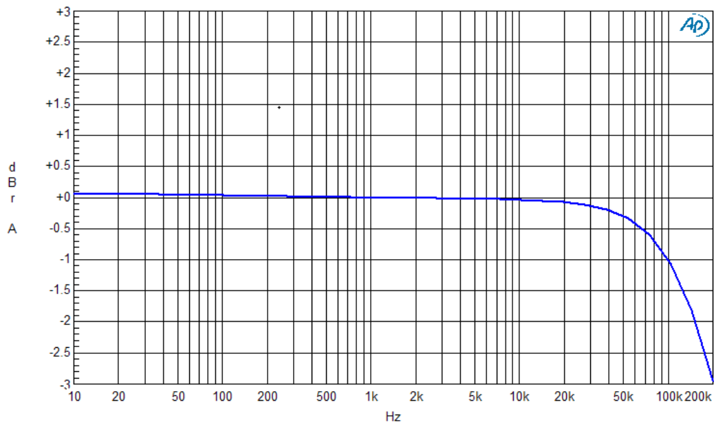
1W-Frequenzgang rechter und linker Kanal
