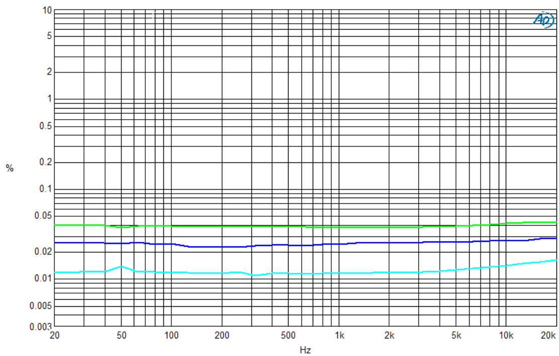
T.H.D + N gegen die Frequenz auf 8 \Omega Klasse A, 80 kHz Messband (1W BLAUE Kurve, 10W HELLBLAUE Kurve und 40W GRÜNE Kurve)
