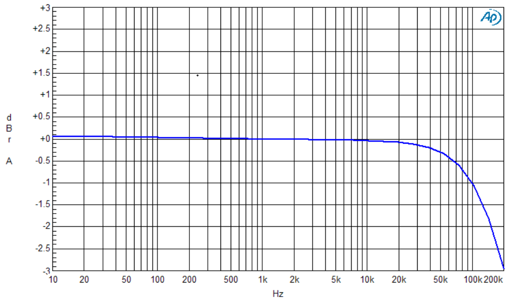
Réponse en fréquence à 1W canal gauche et droit
