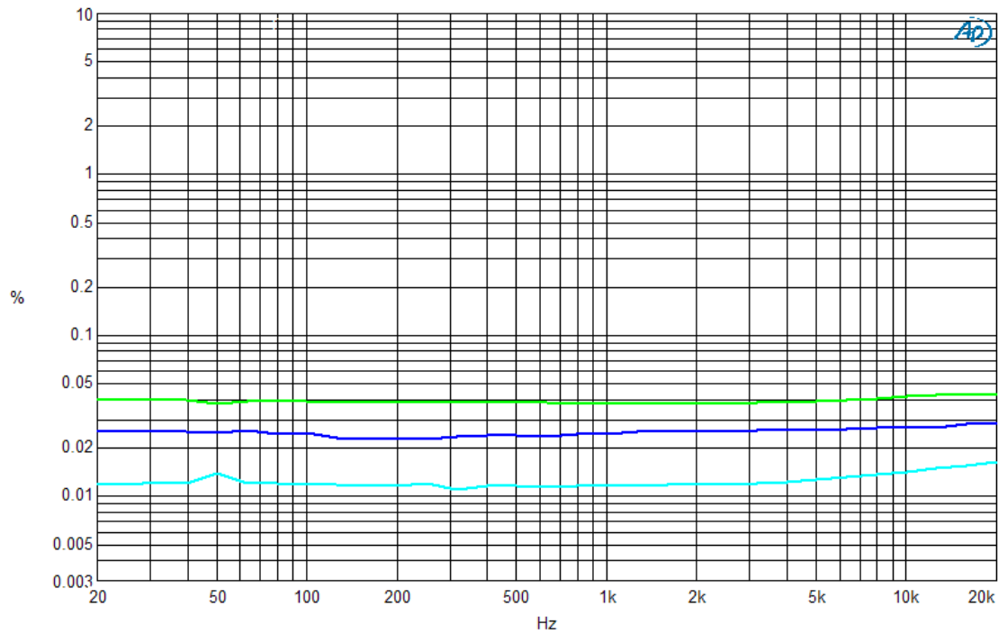
T.H.D + N par rapport à la fréquence sur 8Ω classe A, 80kHz bande de mesure. (1W courbe BLEU, 10W courbe BLEU CLAIR et 40W courbe VERTE)
