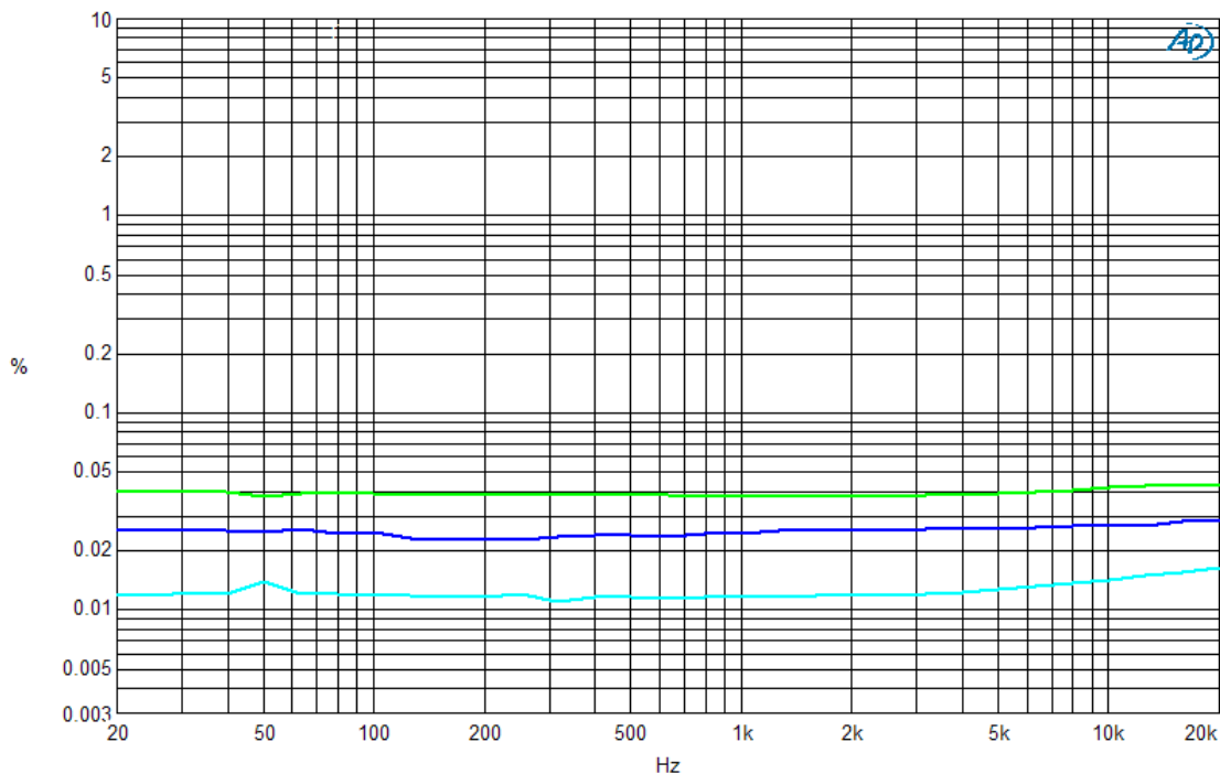
T.H.D + N rispetto alla frequenza su 8Ω classe A, 80kHz banda di misura. (1W curva BLU, 10W curva CELESTE e 40W curva VERDE)
