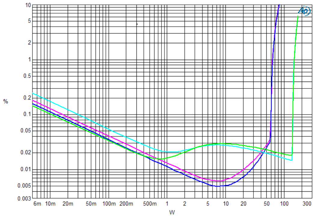
T.H.D + N gegen Ausgangsspannung auf 8 \Omega Klasse A und Klasse AB, 22 kHz Messband (BLAU Kanal L Klasse A, PINK Kanal R Klasse A, GRÜN Kanal L Klasse AB, HELLBLAU Kanal R Klasse AB)
