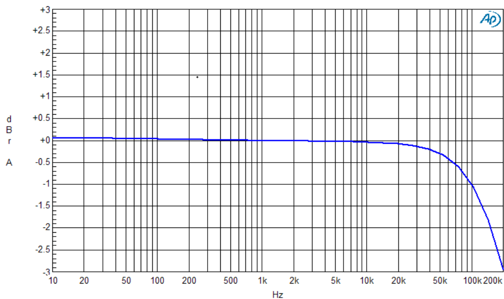
Risposta in frequenza a 1W canale destro e sinistro
